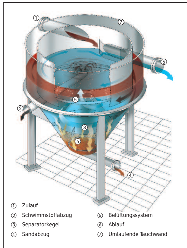
Prinzipische Skizze des HUBER Rundsandfanges HRSF
