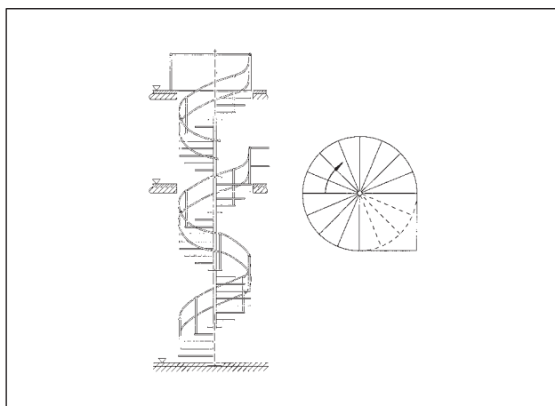
GE 9 Вита стълба
