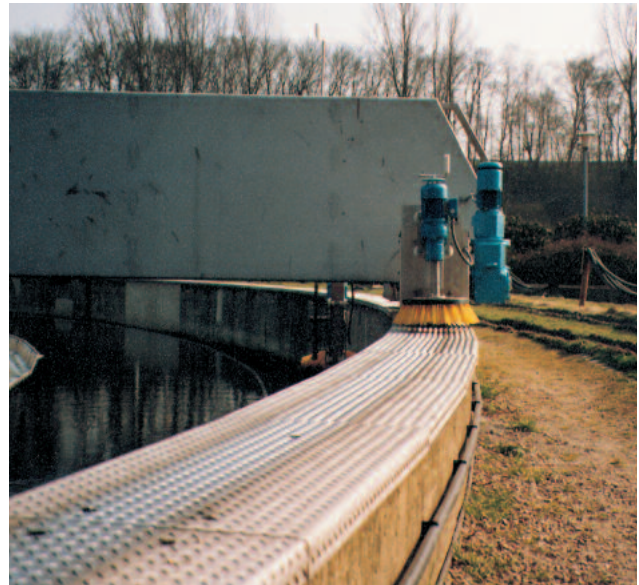
Beckenkronenabdeckung für Rundbecken aus Edelstahl-Tränenblech
