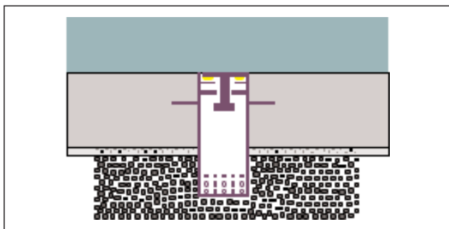
Клапан за подпочвени води КА 6
