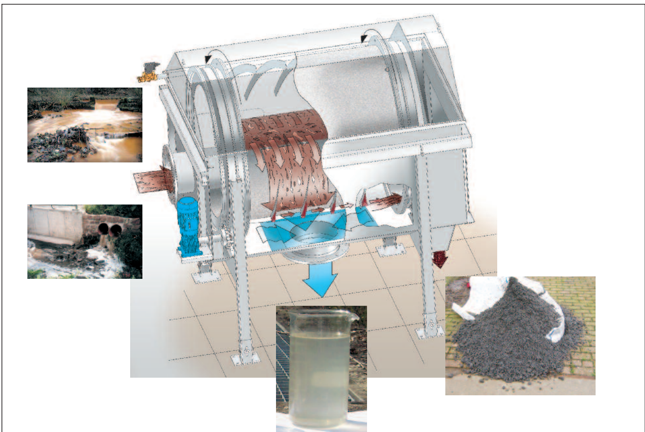
Prinzipdarstellung des HUBER Trommelsiebes RoMesh®
