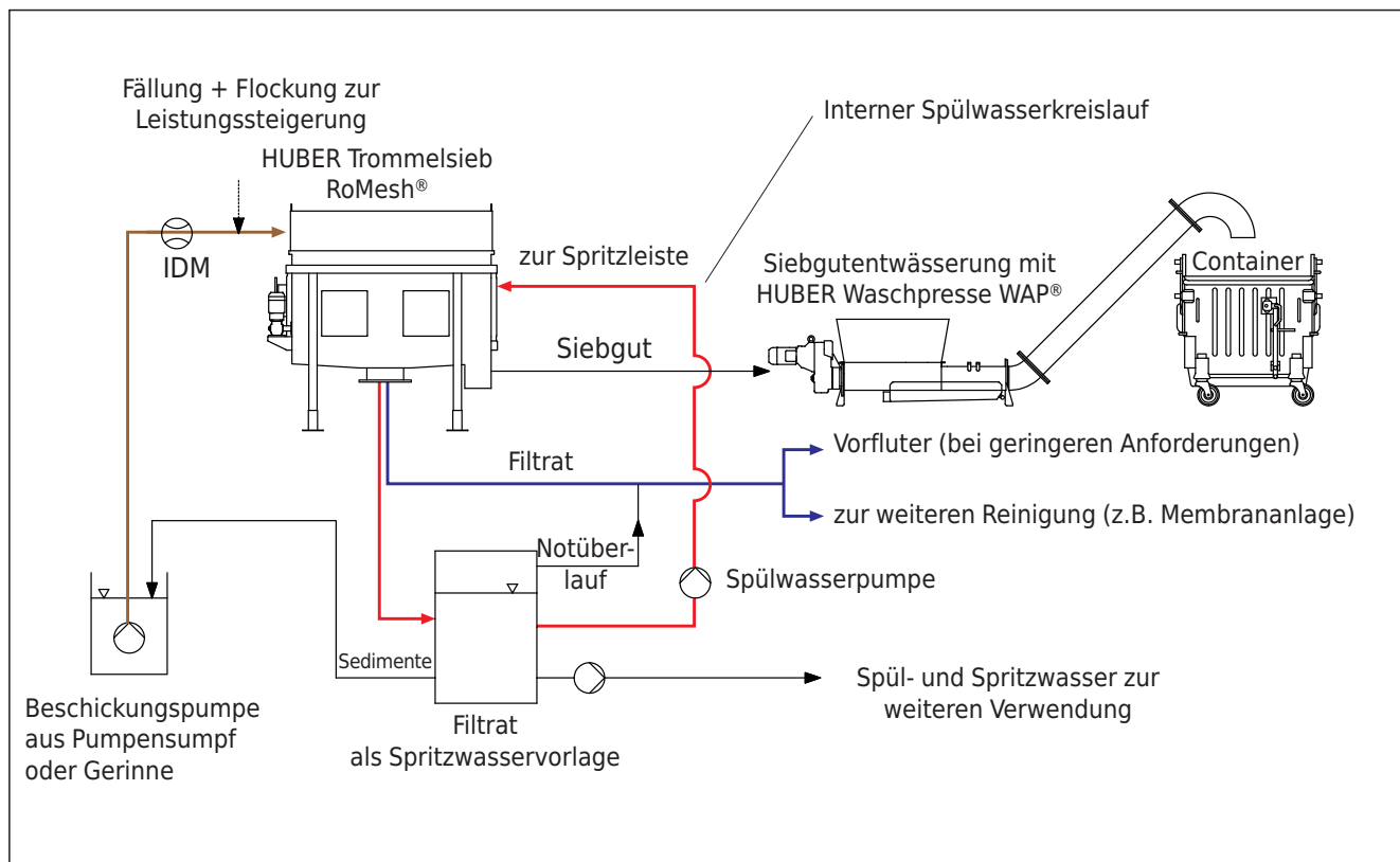
Fließbild einer mechanischen Abwasserreinigung mittels HUBER Trommelsieb RoMesh®
