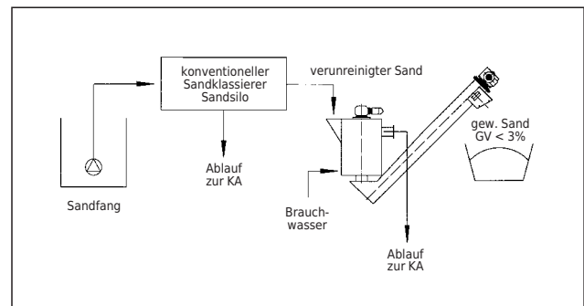
Verfahrensschema
