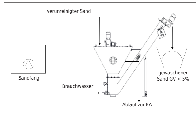
Verfahrensschema
