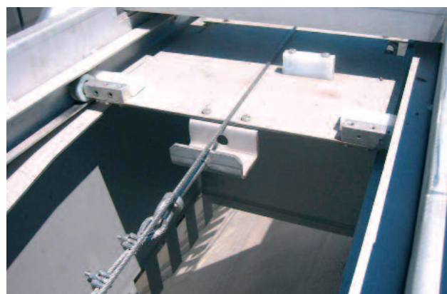
Automatische Fetträumung mittels Fettpaddel
