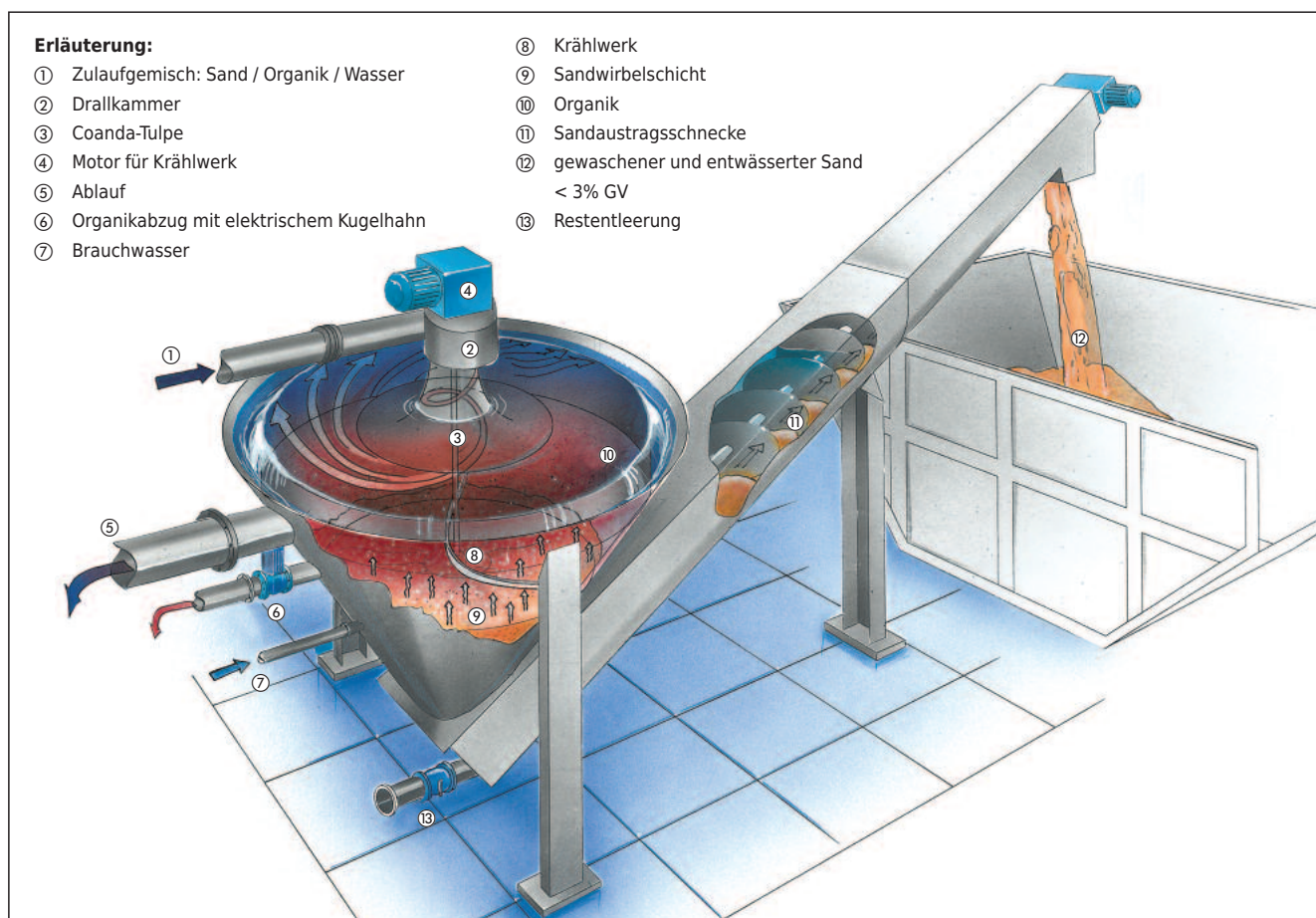
Prinzipische Skizze der HUBER Coanda Sandwaschanlage RoSF4
